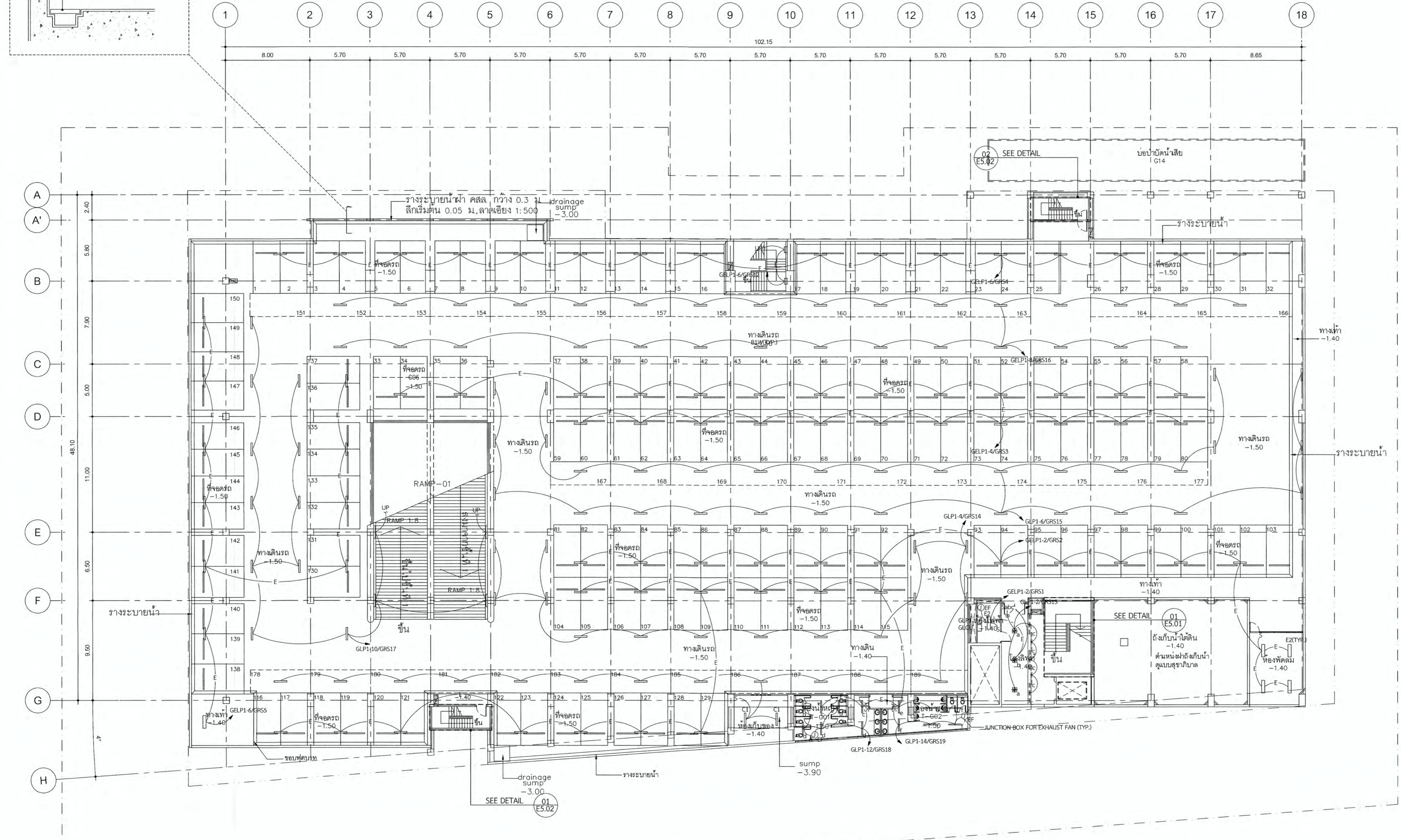
ผังระบบไฟฟ้าแสงสว่าง ชั้นล่าง SCALE 1 : 200
