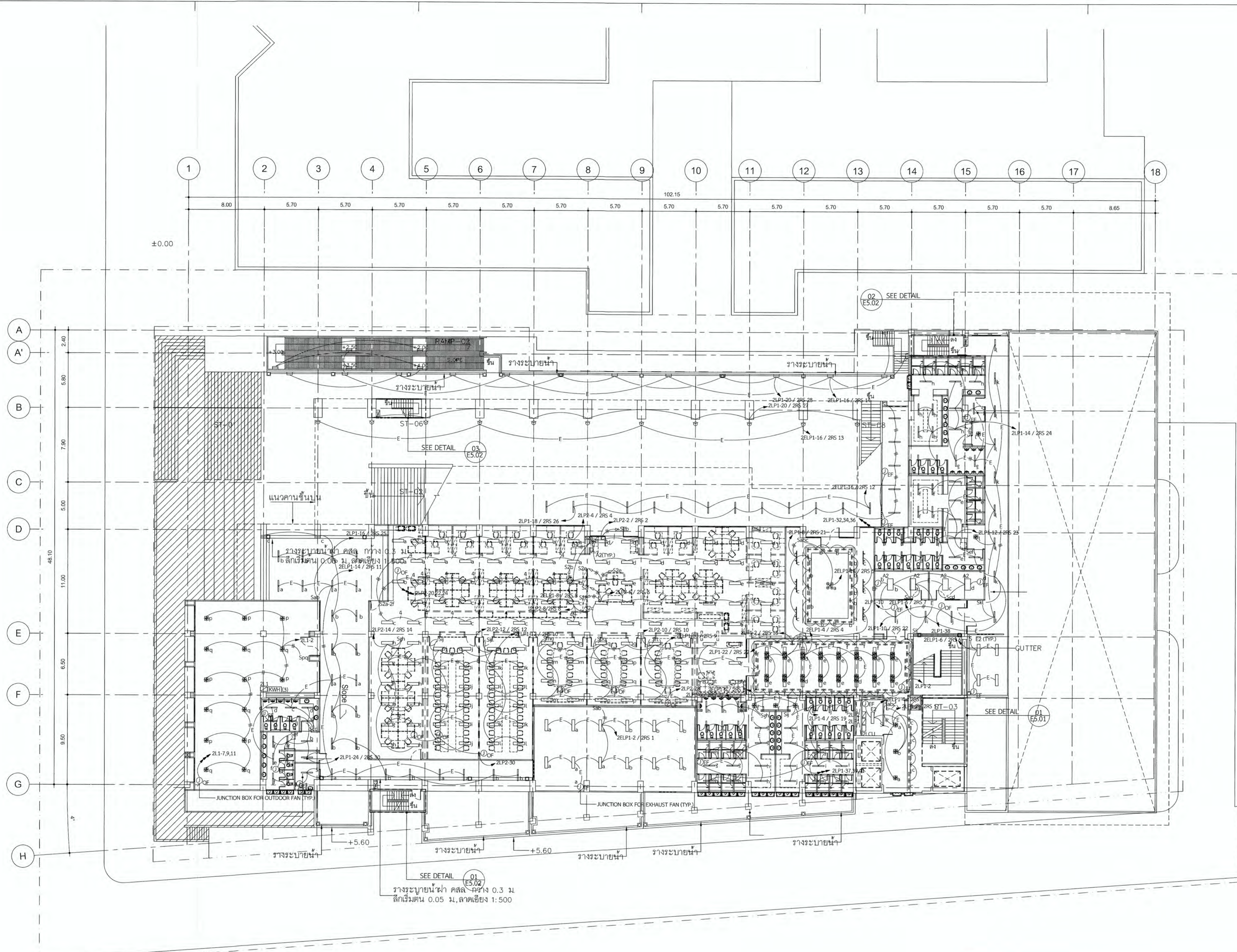
ผังระบบไฟฟ้าแสงสว่าง ชั้นที่ 2 SCALE 1:200
